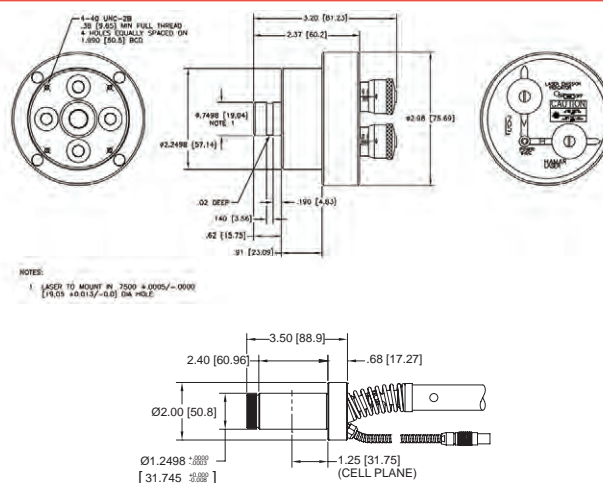
A-512 2-Axis Target
